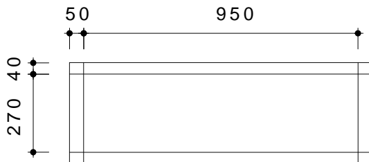
平面図（脚）
